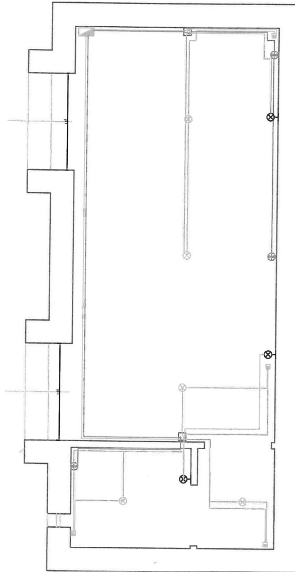
Planimetria impianti elettrici
