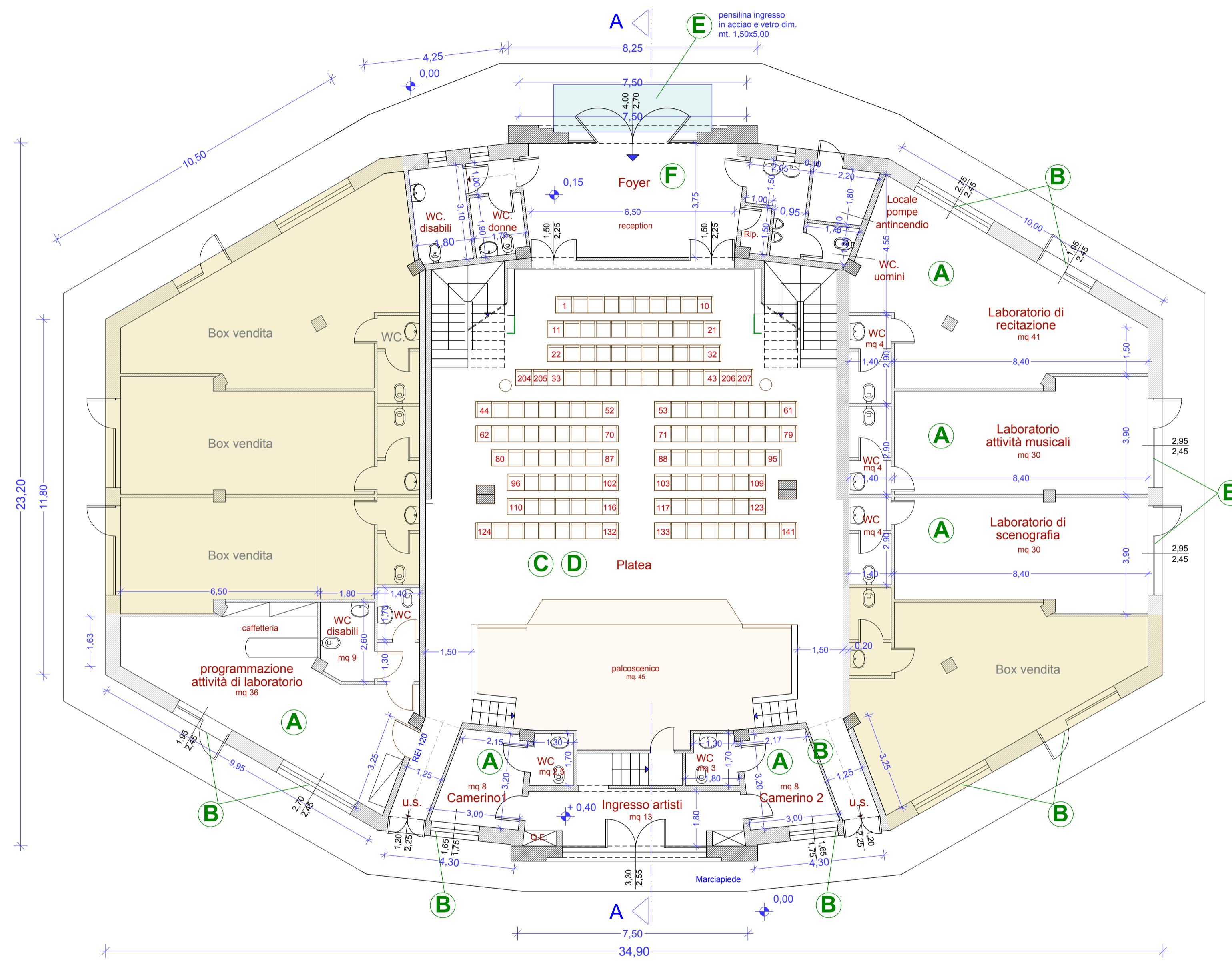
PIANTA A QUOTA +1,50 scala 1:100
