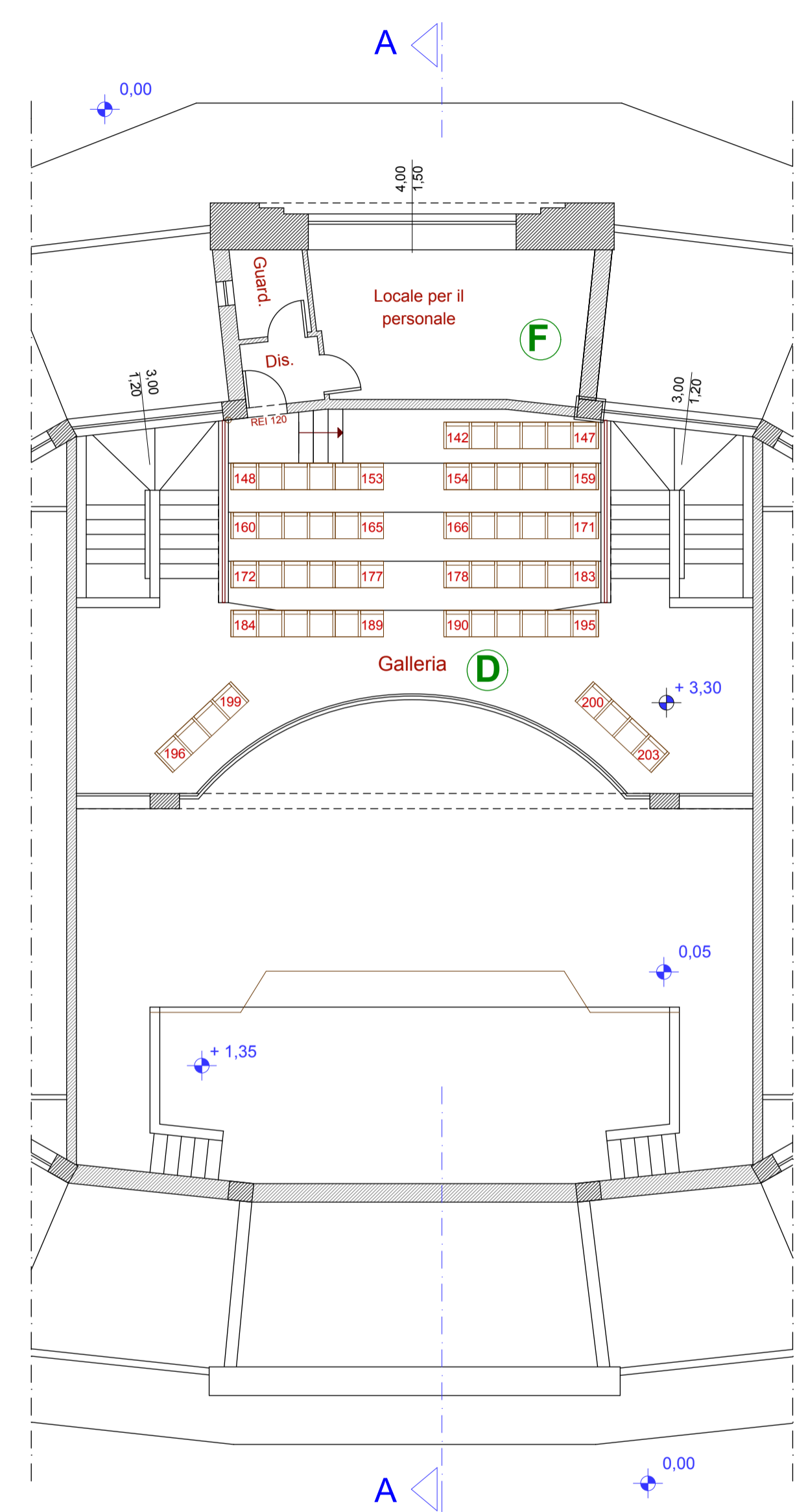
PIANTA A QUOTA +5,00 scala 1:100
