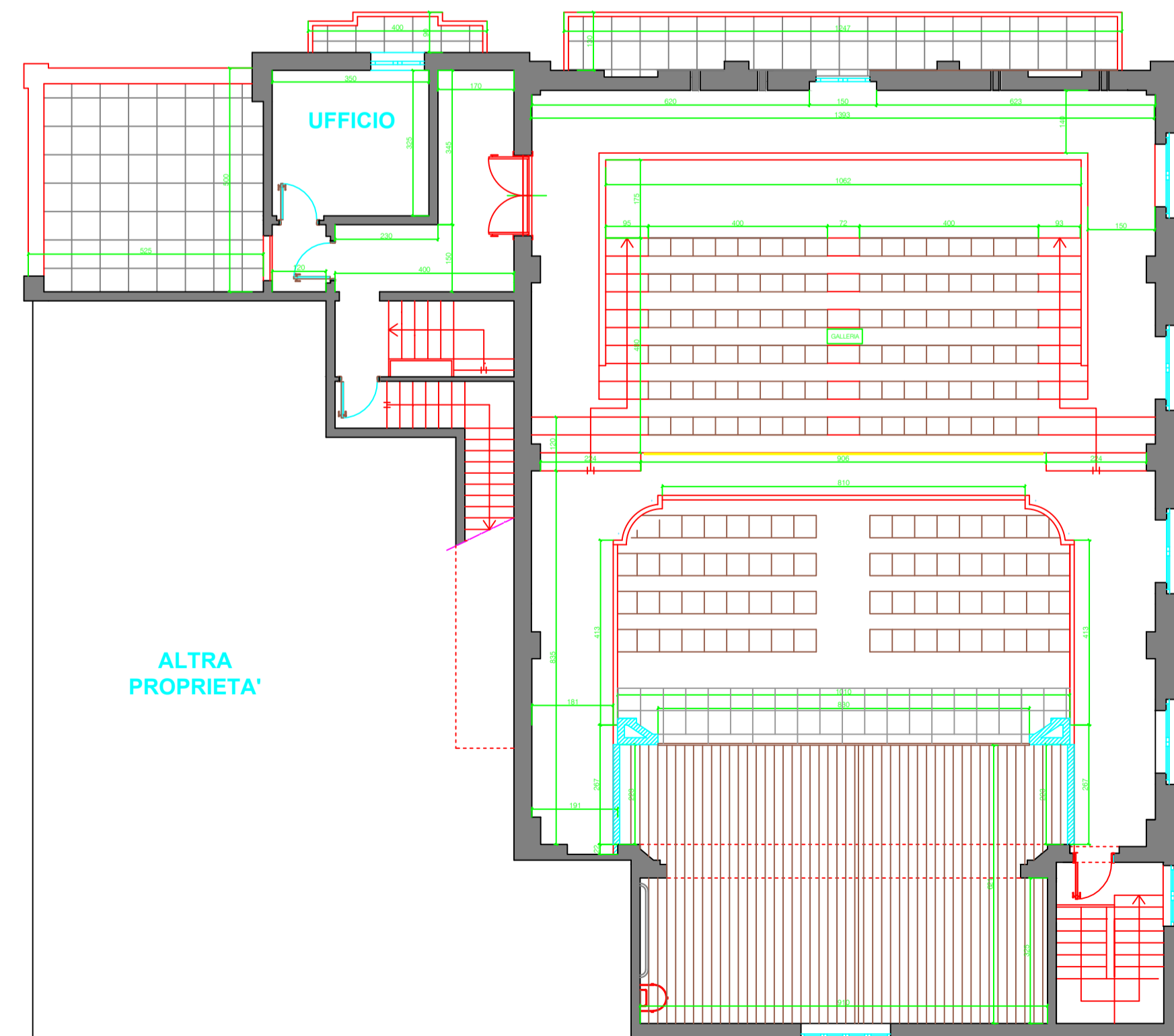
Pianta piano primo - galleria
