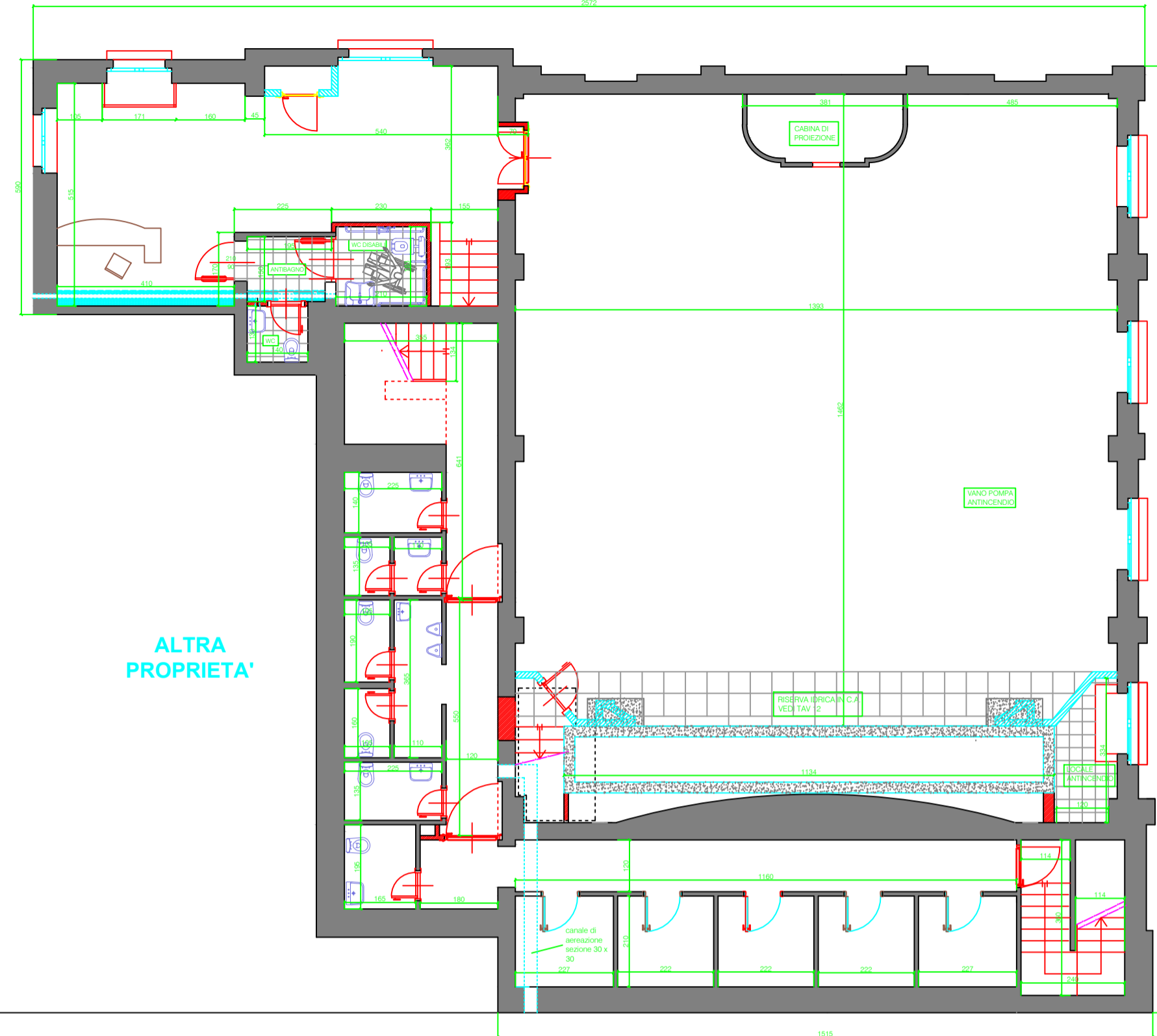
Pianta piano interrato - sottopalco
