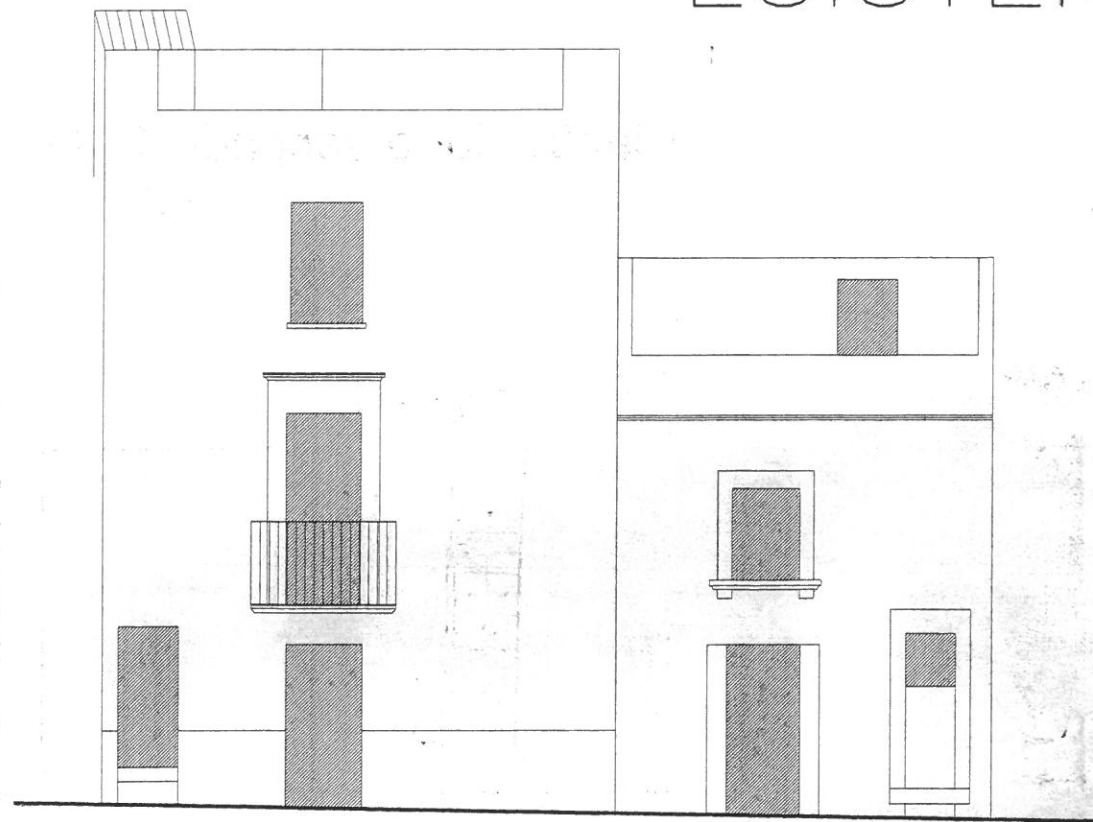
Prospetto 1:100
