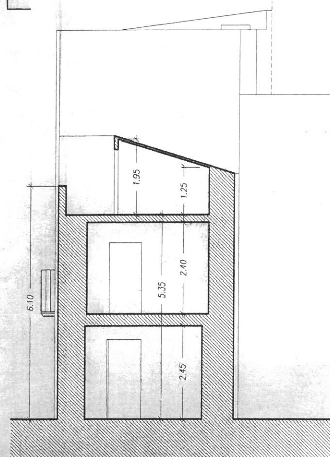
Sezione CD 1:100
