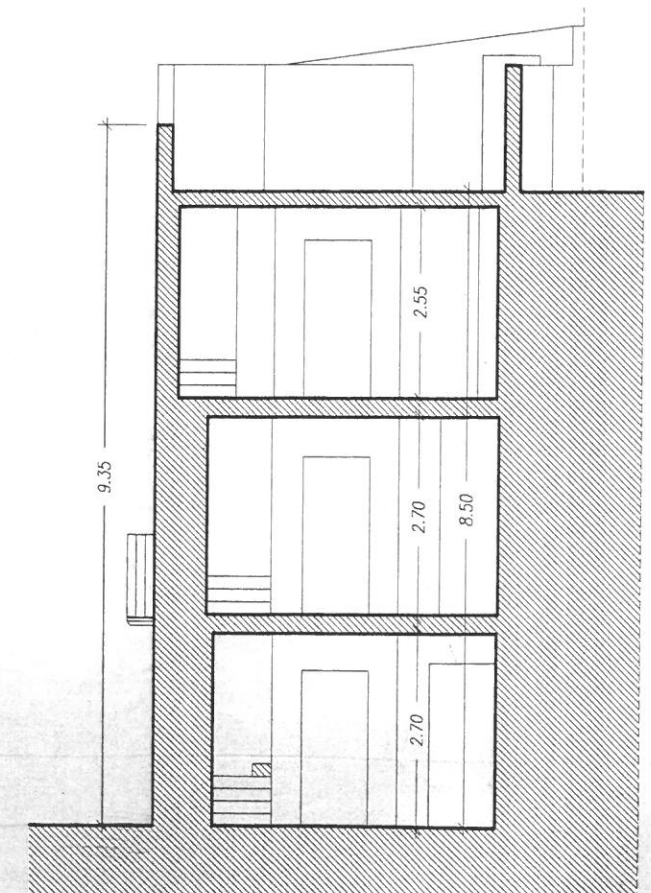
Sezione AB 1:100
