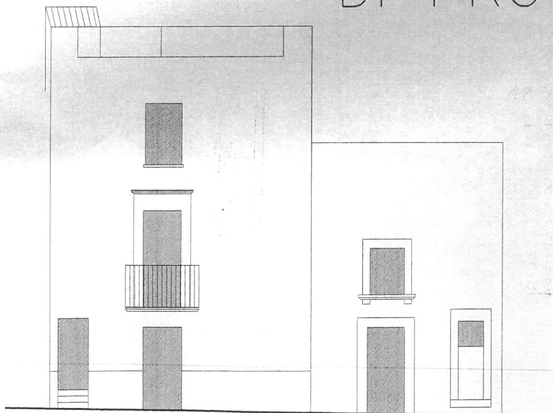
Prospetto 1:100
