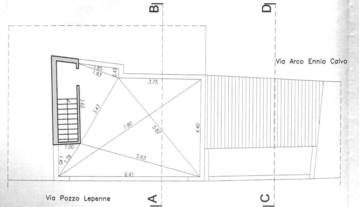
Pianta piano copertura 1:100
