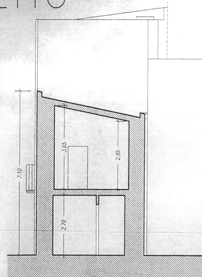
Sezione CD 1:100
