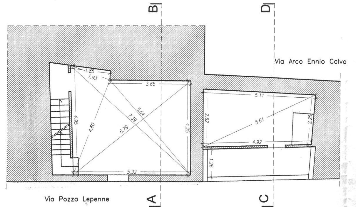
Pianta piano secondo 1:100
