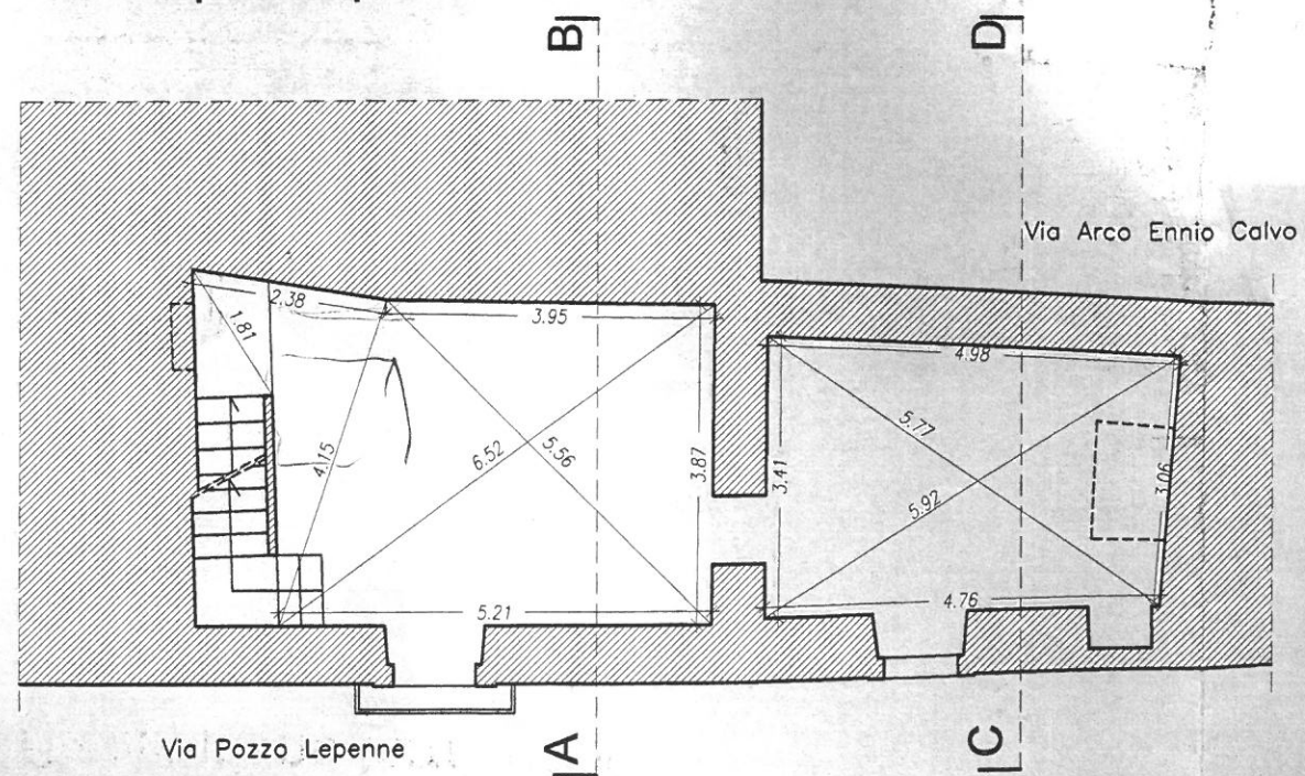
Pianta piano primo 1:100
