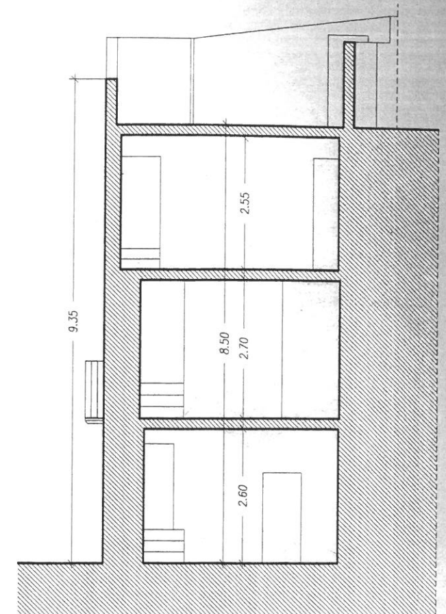
Sezione AB 1:100
