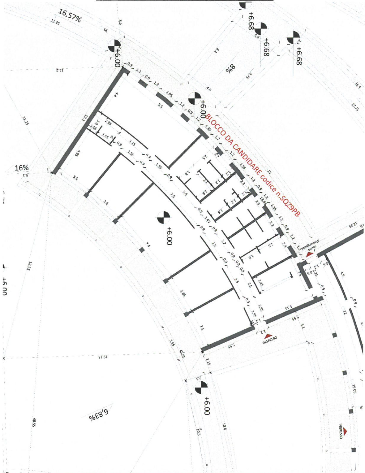
PIANTA QUOTATA
