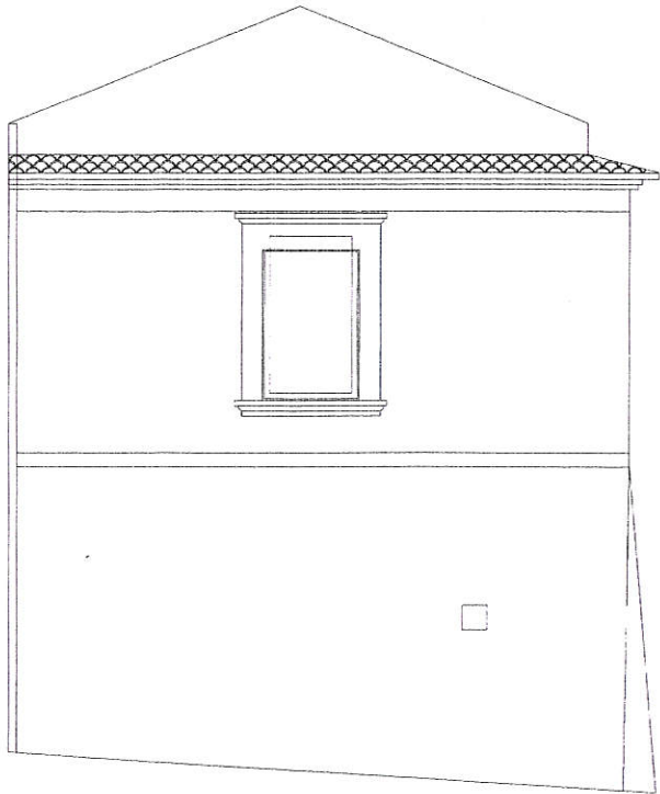
PROSPETTO SU VIA MAUREA - RILIEVO
